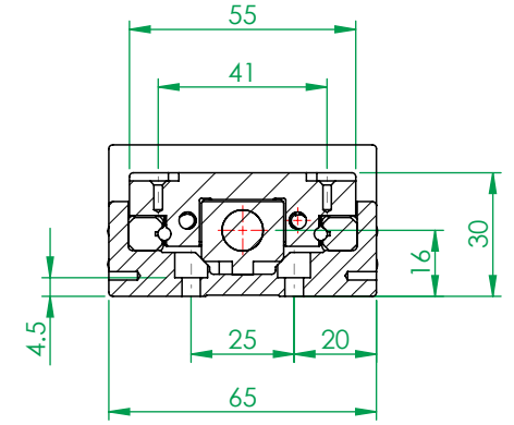
剖面圖 K-K
